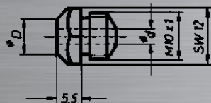
Стандартная насадка
