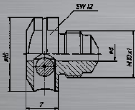
Пружинная насадка
