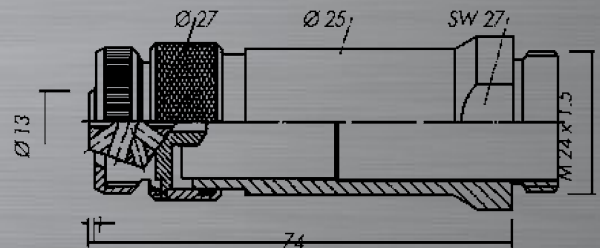
Универсальная насадка
